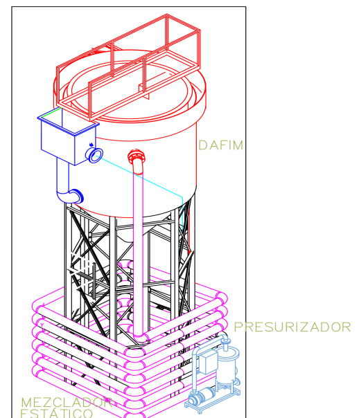
DIBUJO DEL EQUIPO COMPLETO
