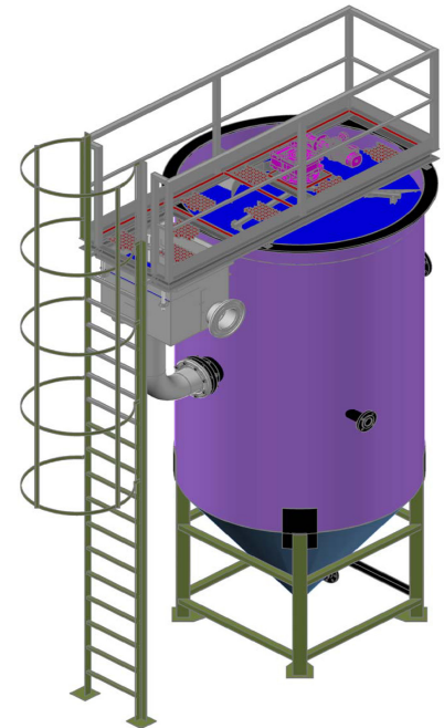
Figura 1: Diseño 3D del DAFIM
